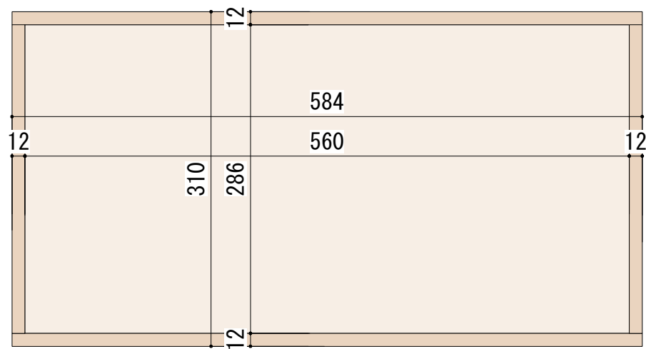
木箱平面図
