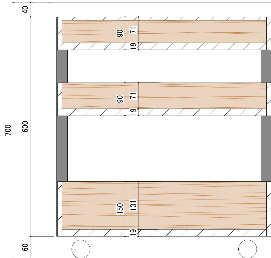
段面図 (1)
