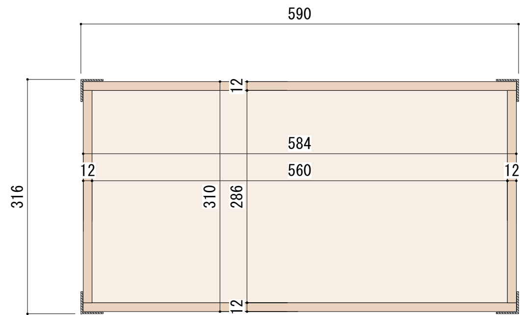
平面図
