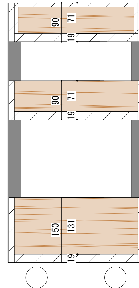
段面図 (2)
